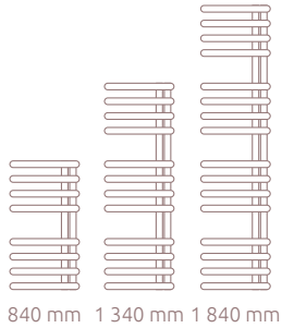
Nákresy výškových variánt:
