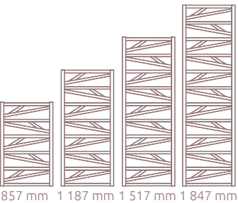
Nákresy výškových variánt:
